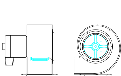
AMU 75 – AMU 400
